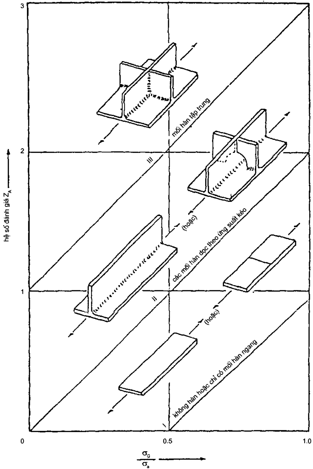
Hình 3.1. Z_A theo các điều kiện của ứng suất và môi hàn
