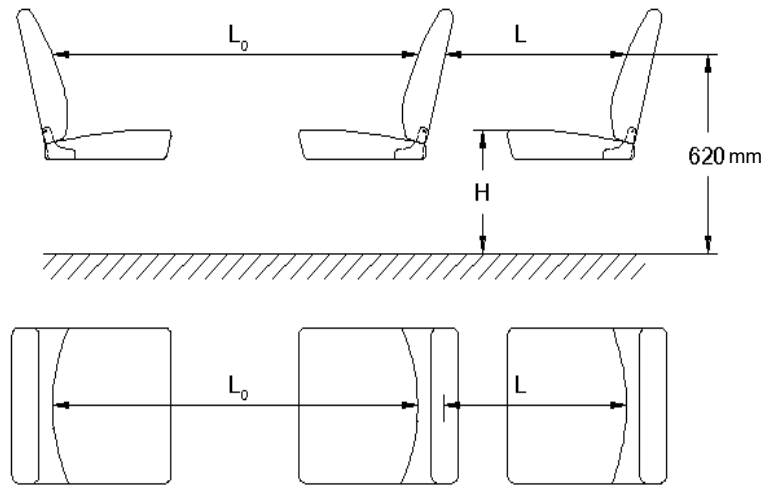
Hình 2 - Kích thước giữa các ghế
