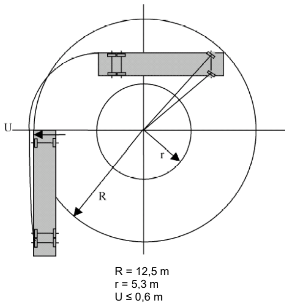
Hình 6a - Khả năng quay vòng xe thân liền
