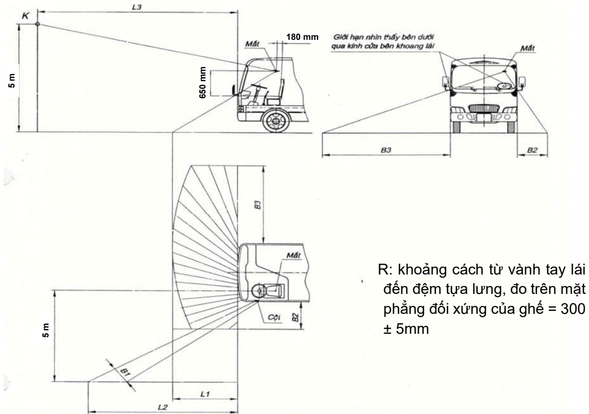
Hình 1 - Tầm nhìn của người lái
