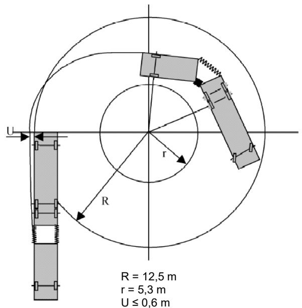
Hình 6b - Khả năng quay vòng xe nối toa
