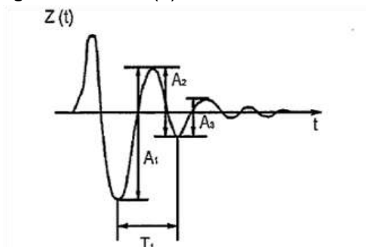
Hình 1-2a - Đường cong dao động tắt dần của thân xe.
